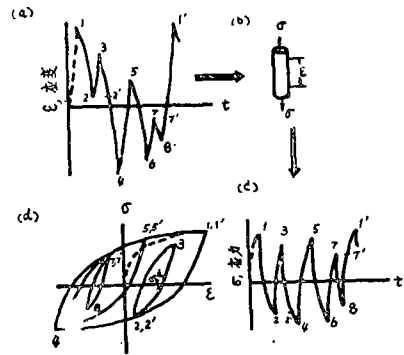
图2 施加在光滑试件上的应变-时间历史和应力响应
