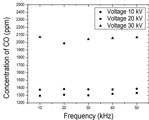
图3 出口CO浓度与电压、频率的关系
