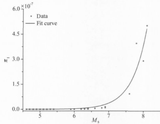
图 3 \pi_1 与震级的关系
