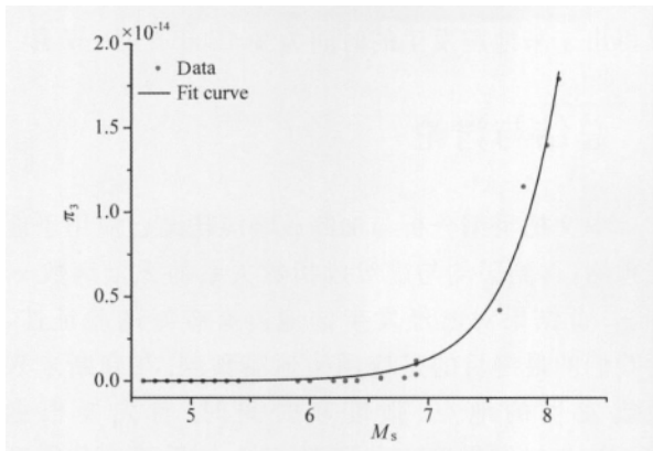
图 4 \pi_3 与震级之间的关系
