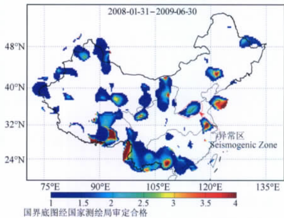
图 6 河南周口地震异常区(图中红色连线包围的区域)
