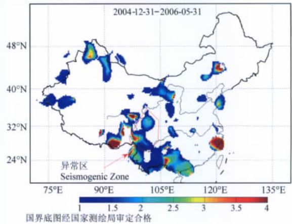
图 5 汶川地震(2008)加卸载响应比异常区(图中红色连线包围的区域)
