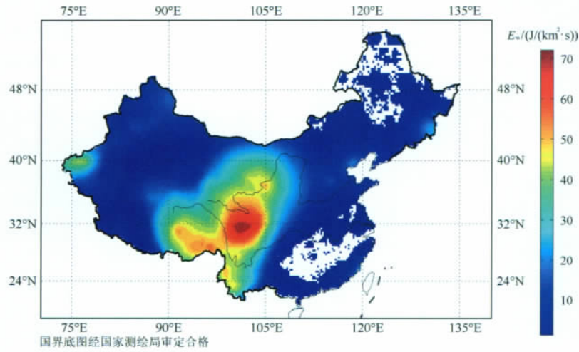
图 1 中国陆地各地平均地震波能量 E_w 的分布图
